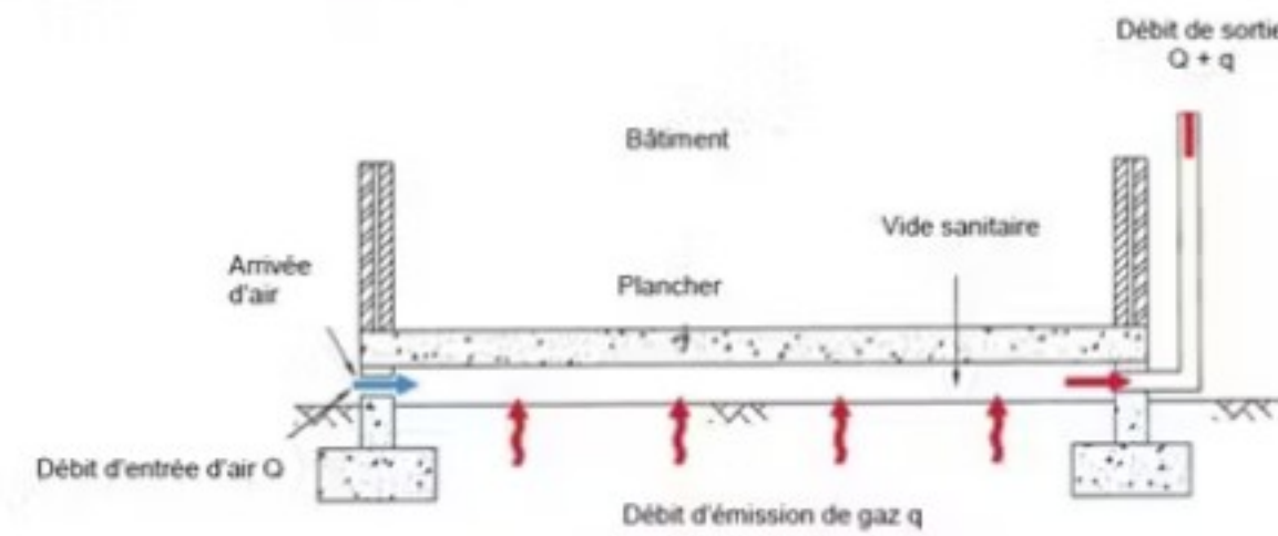
Figure 10 : Principe de la ventilation d'un vide sanitaire [18].
